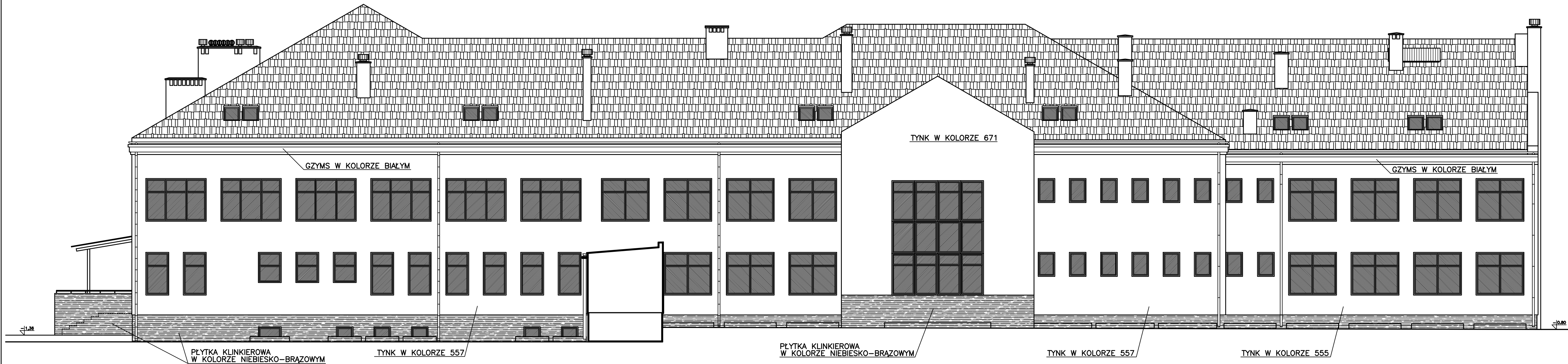
ELEWACJA PÓŁNOCNO-ZACHODNIA SKALA 1:100
